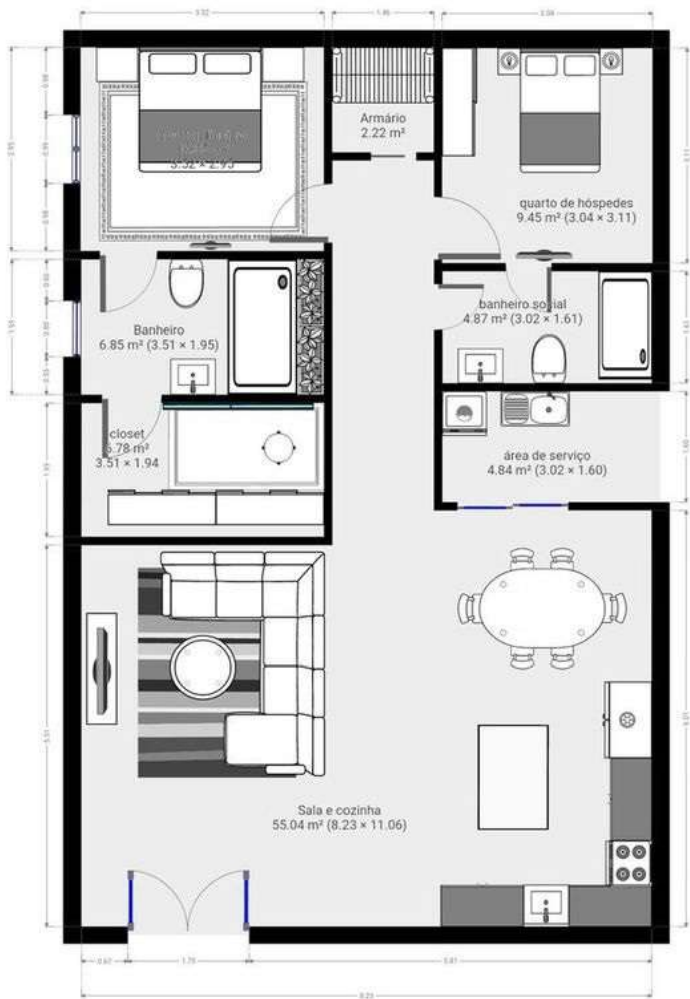
PLANTA BAIXA
